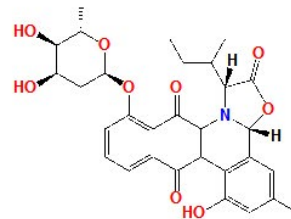
jadomycin B (24)
