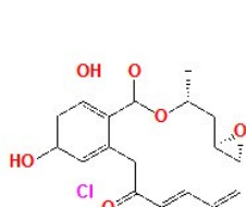
dradicicol (22)
