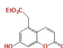
quadrisepin A (21)
