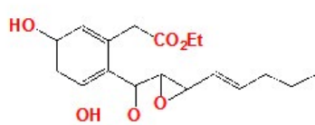
cytosporone I (19)
