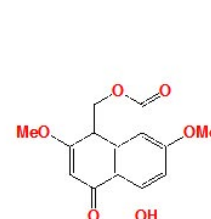
corymbiferone (25)
