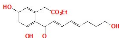
cytosporone G (17)
