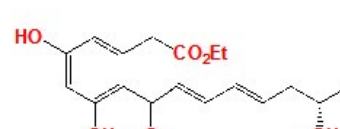
cytosporone H (18)
