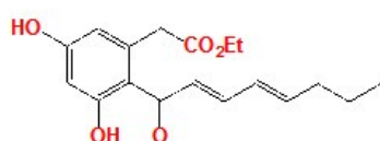
cytosporone F (16)
